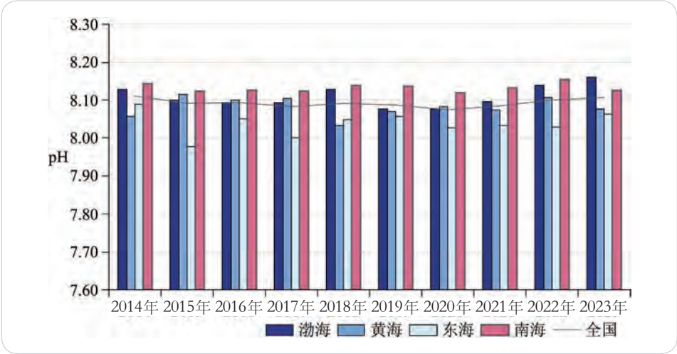
2014-2023 年夏季我国近岸海域表层海水 pH
