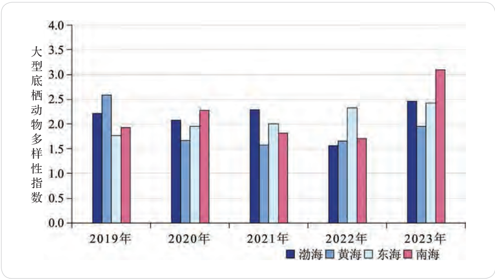
2019-2023 年夏季我国近岸海域大型底栖动物多样性指数
