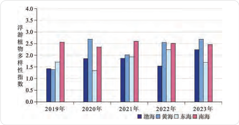
2019-2023 年夏季我国近岸海域浮游植物多样性指数
