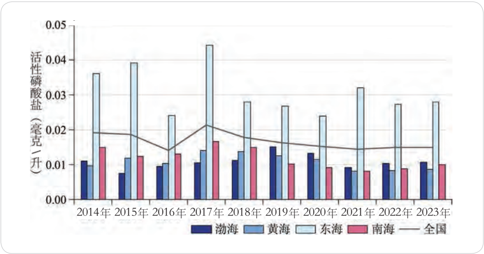
2014-2023 年夏季我国近岸海域海水中活性磷酸盐浓度
