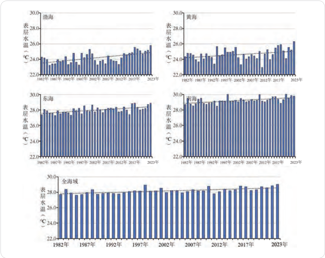
1982-2023 年夏季我国近海表层水温 (左上：渤海；右上：黄海；左中：东海；右中：南海；下：全海域)
