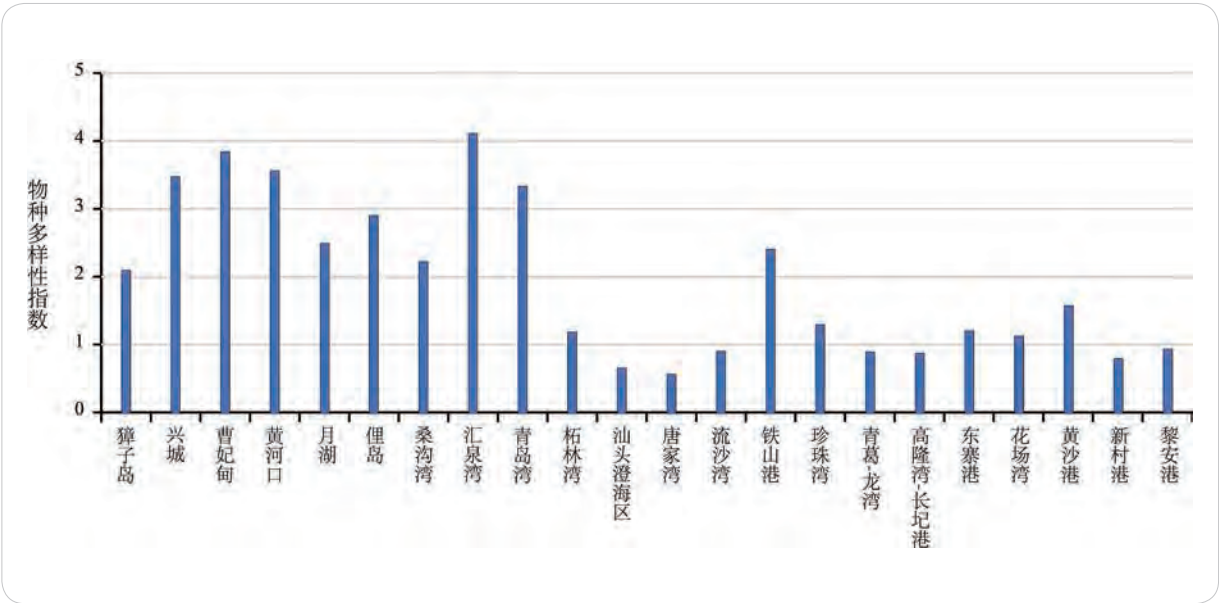
2020 年 22 个主要调查区域大型底栖动物物种多样性指数
