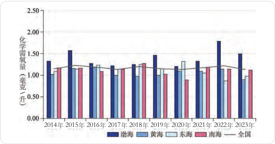
2014-2023 年夏季我国近岸海域海水化学需氧量浓度
