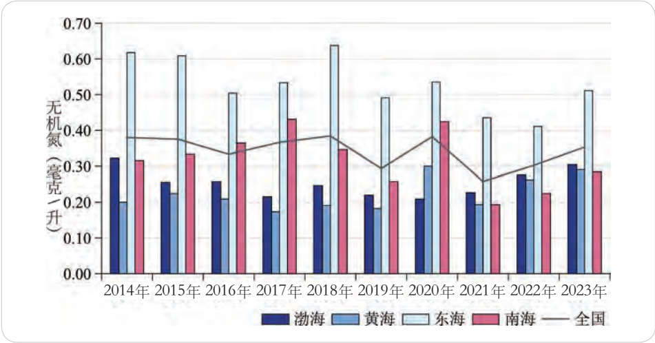
2014-2023 年夏季我国近岸海域海水中无机氮浓度
