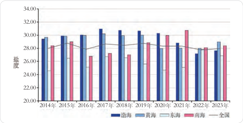
2014-2023 年夏季我国近岸海域表层海水盐度
