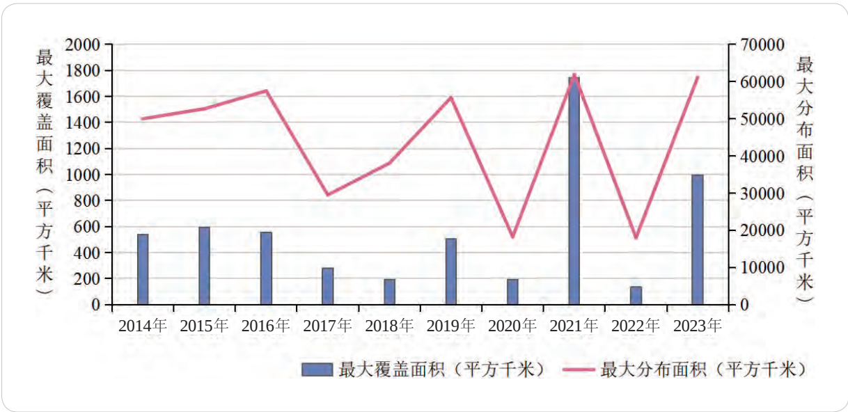
2014-2023 年我国黄海浒苔绿潮年度规模
