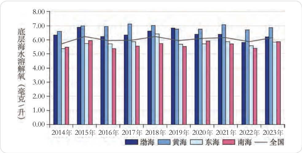
2014-2023 年夏季我国近岸海域底层海水溶解氧浓度
